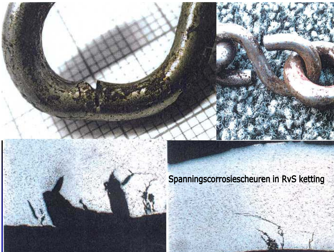
Voorbeeld van spanningscorrosie in kettingen uit een zwembad
