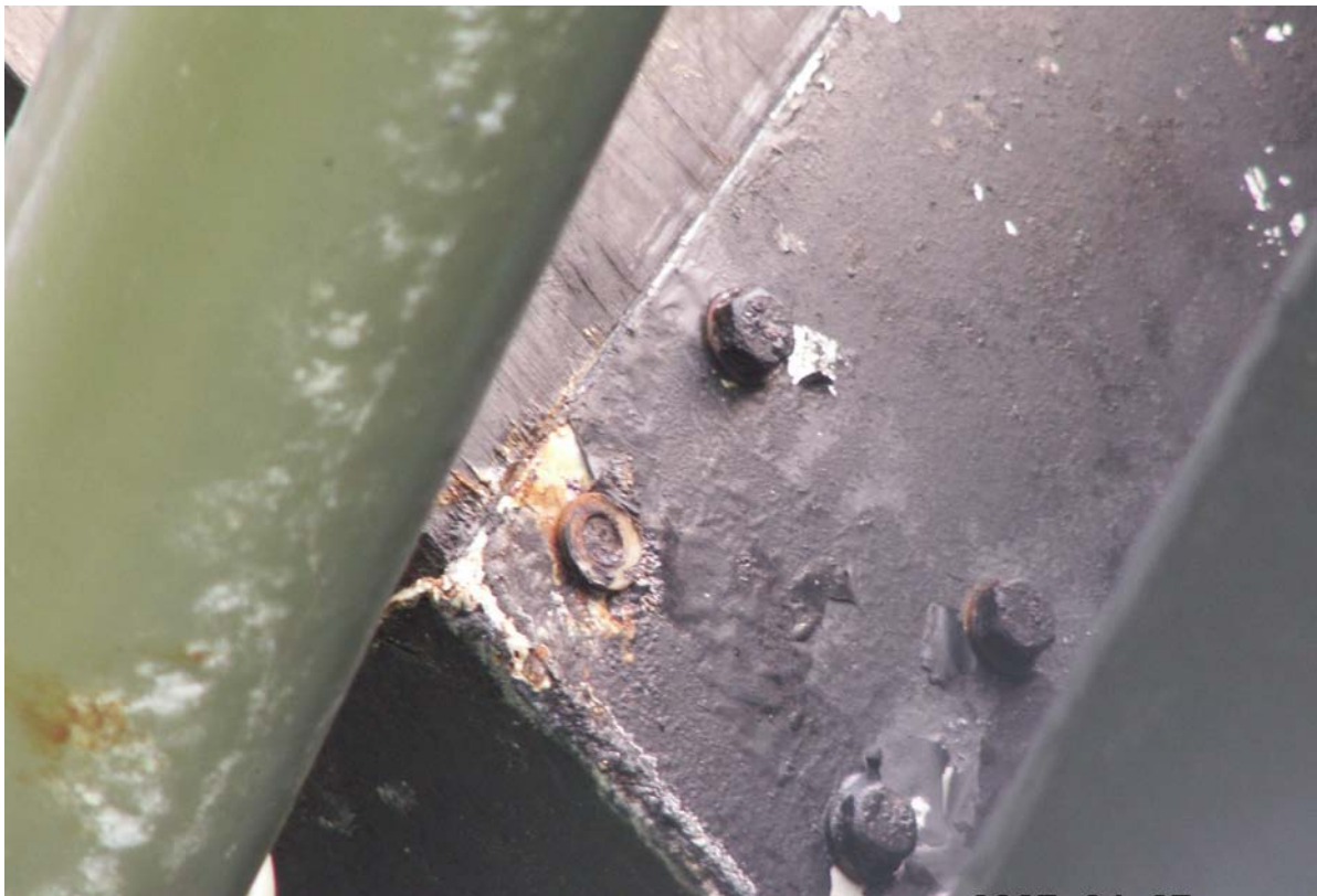
He, nog een kop van een bout verdwenen vanaf ca 20 meter hoogte
