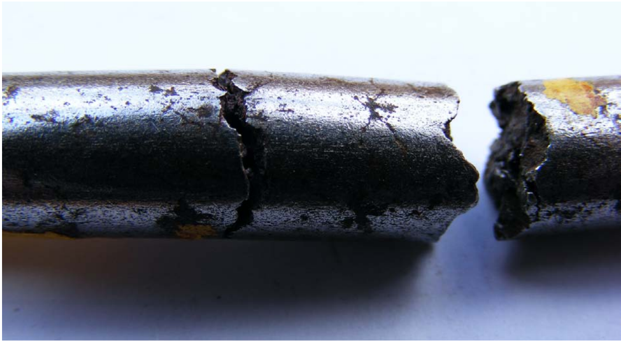
Gebroken Roestvaststalen bout tengevolge van spanningscorrosie
